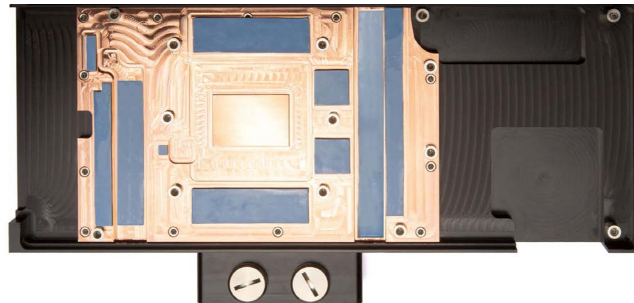
Kühler mit Wärmeleitpads Cooler with thermal pads
